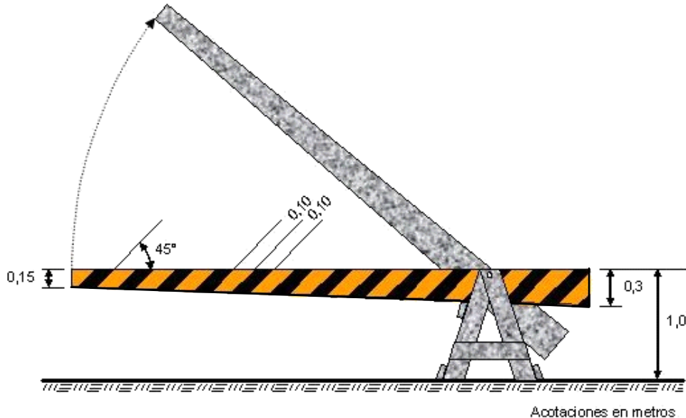
FIGURA 1.- Barrera levadiza
